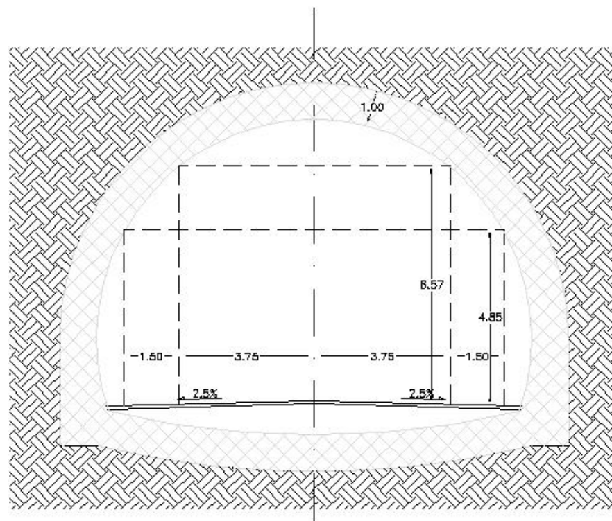
Sezione tipo in galleria
